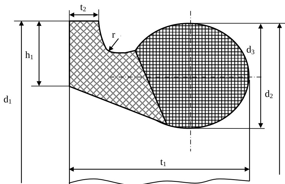
Рисунок 2.3 Уплотнительное резиновое кольцо типа «TYTON».
