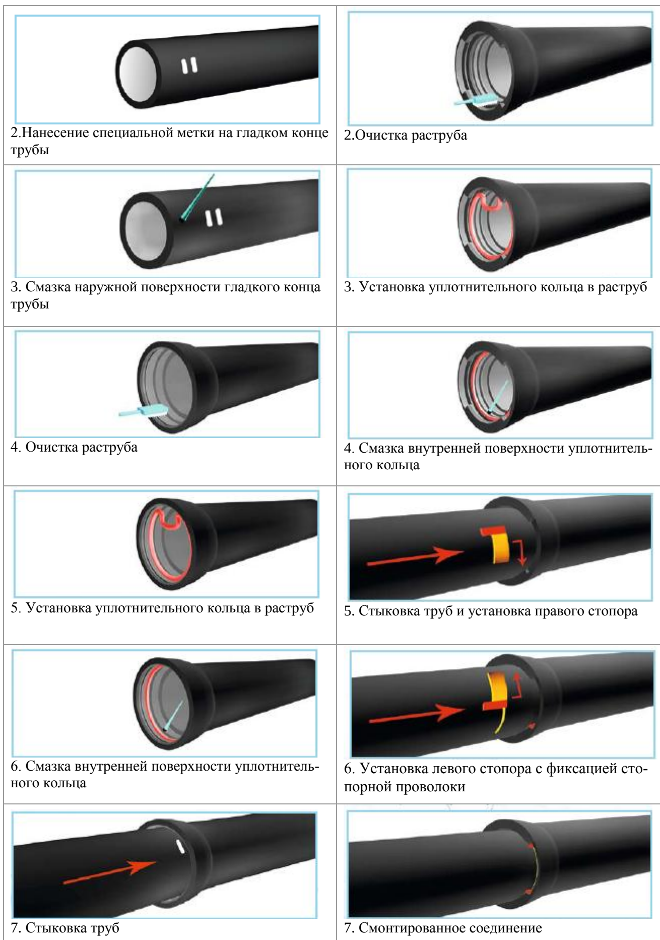
Рисунок 6.5 Монтаж труб с соединением TYTON и RJ.
