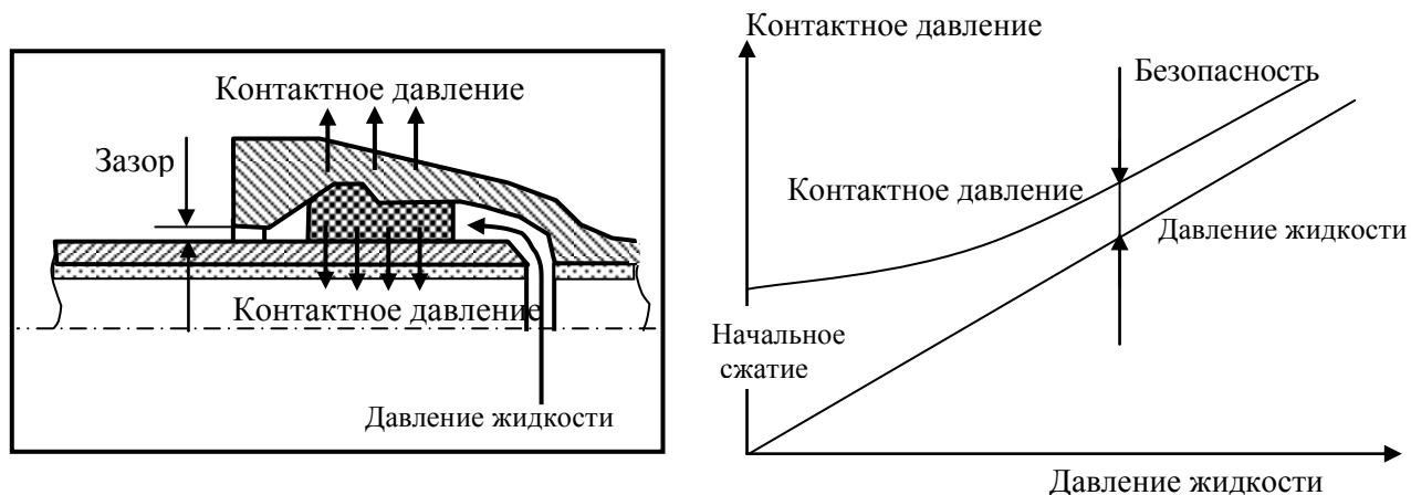
Рисунок 2.16 Контактное давление.
