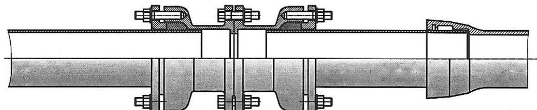
Рисунок 7.6 Ремонт трубопровода при помощи патрубка фланец - раструб компенсационный ПФРК.
