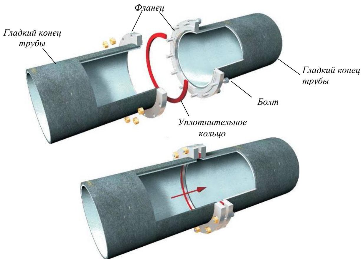
Рисунок 2.12 Фланцевое соединение.
