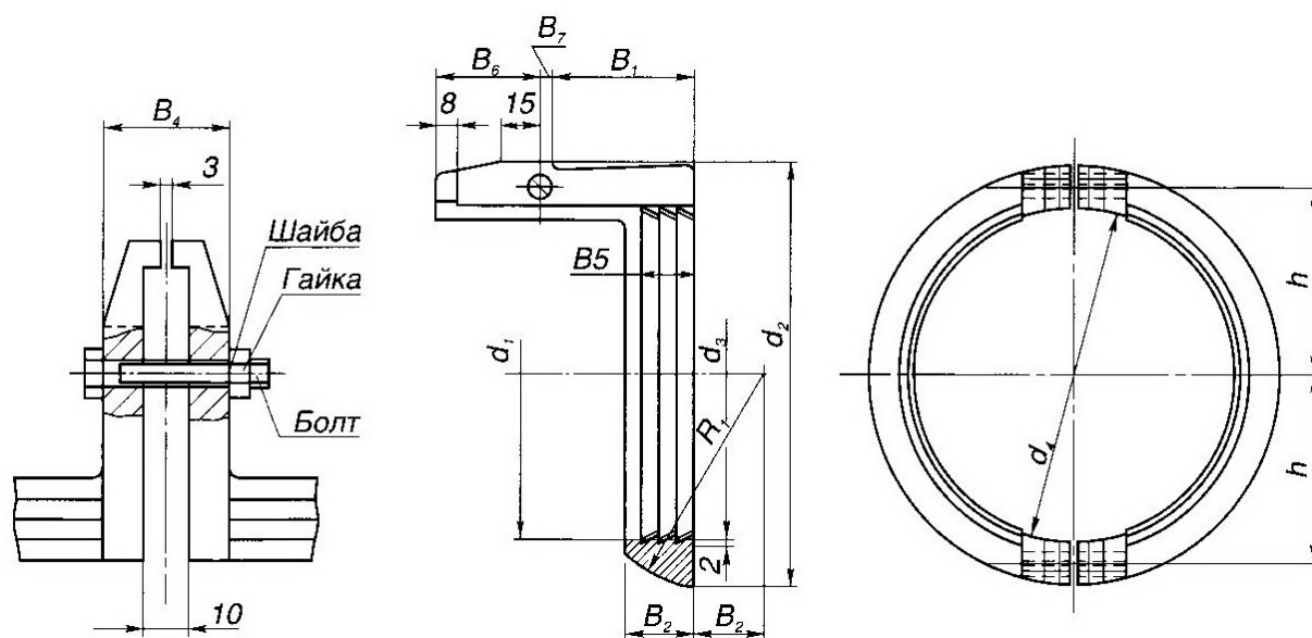
Рисунок 6.11 Стяжное кольцо.
