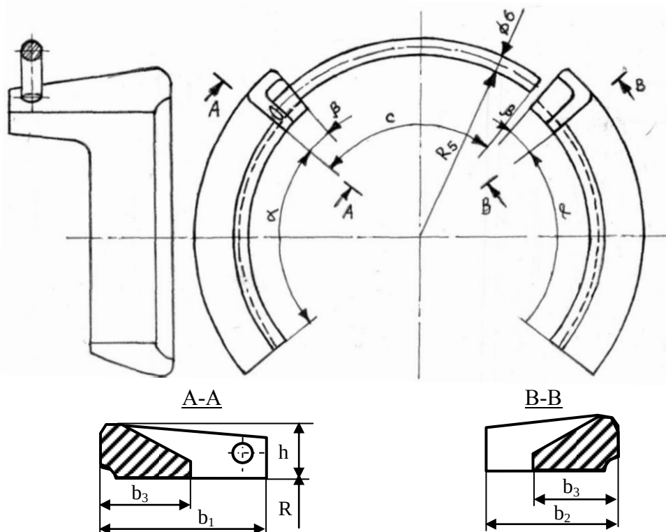
Рисунок 2.8 Стопор из ВЧШГ для соединения «RJ».
