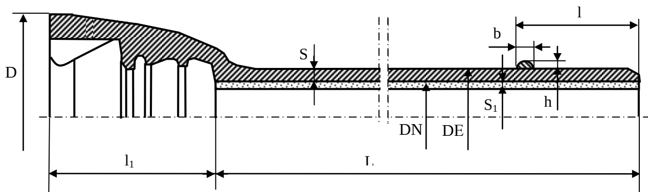
Рисунок 2.6 Труба раструбная с соединением «RJ».
