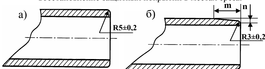
Рисунок 7.3 Торцевой гладкий конец трубы.
