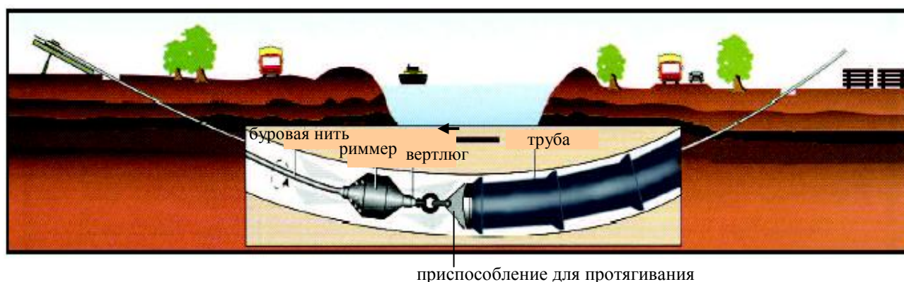
Рисунок 6.20 Протягивание трубопровода.
