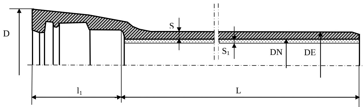
Рисунок 2.2 Труба раструбная с соединением «TYTON».
